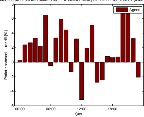
Počet zastavení pro křižovatku 5.601 - Řevnická / Metropole Zličín / Terminal PT (relativní změny)
