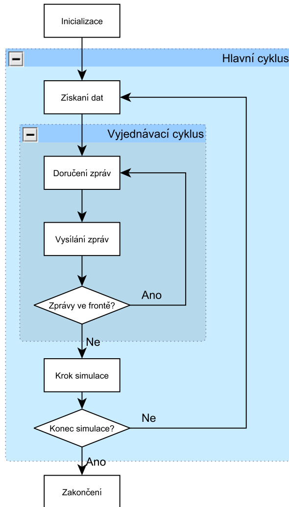
Obrázek 3.4: Struktura fungování programu main_loop.exe , podrobněji popsána v podkapitole 3.6
