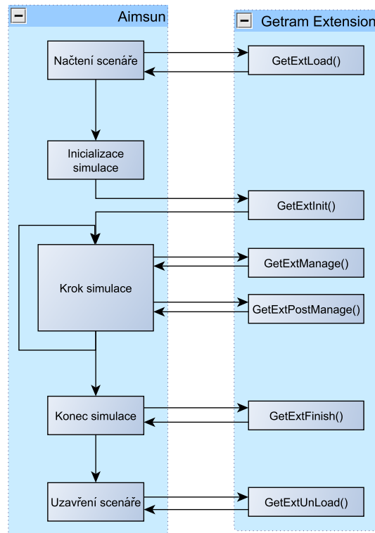
Obrázek 1.6: Podrobný náskres komunikace mezi Aimsunem a Getram Extension.
