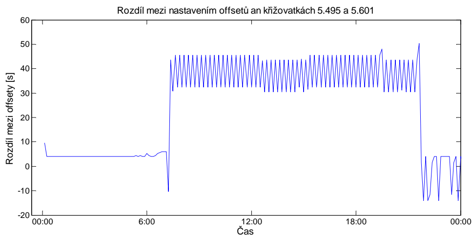
Obrázek 4.3: Rozdíl mezi nastavenými offsety v průběhu simulace s reálnými vjezdy.
