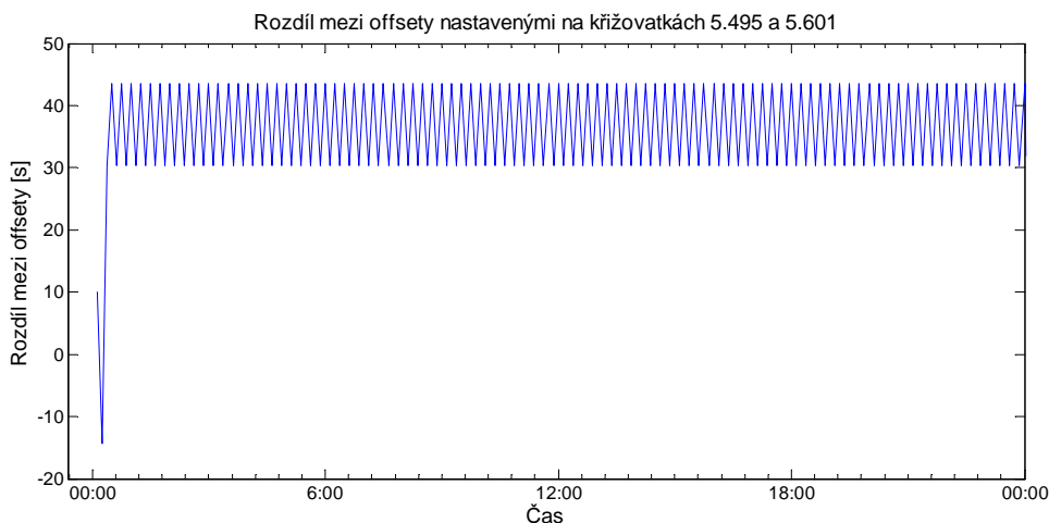
Obrázek 4.1: Rozdíl mezi nastavenými offsety v průběhu simulace s konstantními vjezdy.
