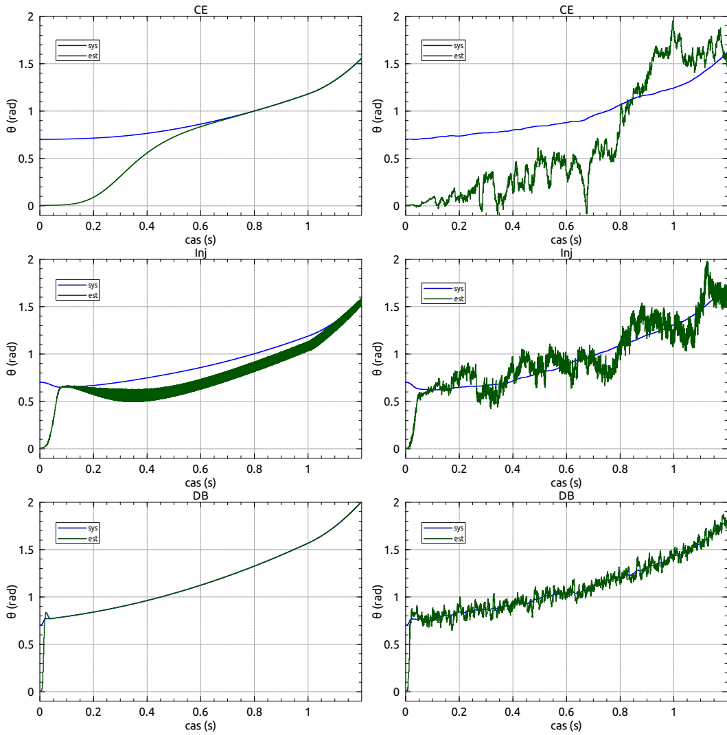
Obrázek 5.5: Porovnání skutečného úhlu natočení \vartheta^{sys} (modrá) s jeho odhadem \vartheta^{est} (zele- lená) pro různé algoritmy při uvažování počáteční hodnoty \vartheta_0^{sys} = \frac{2}{9}\pi . V levém sloupci jsou vždy výsledky bez uvažování šumu ve stroji a šumu měření, v pravém s šumem. Použité algoritmy: nahoře CE, uprostřed jednoduchá injektáž, dole jednoduchý duální přístup.
