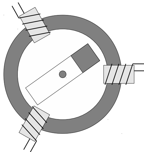
Zjednodušený model PMSM
