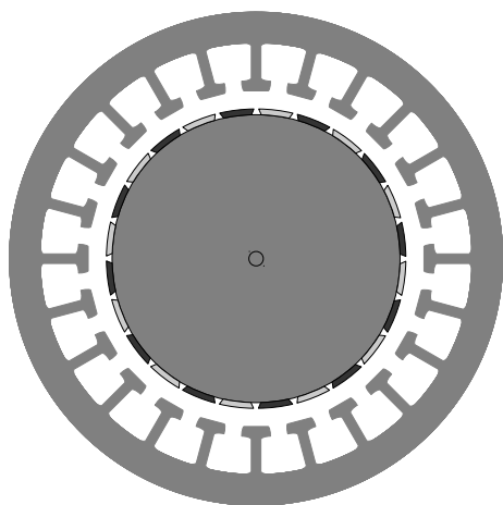
Ilustrativní obrázek konstrukce PMSM
