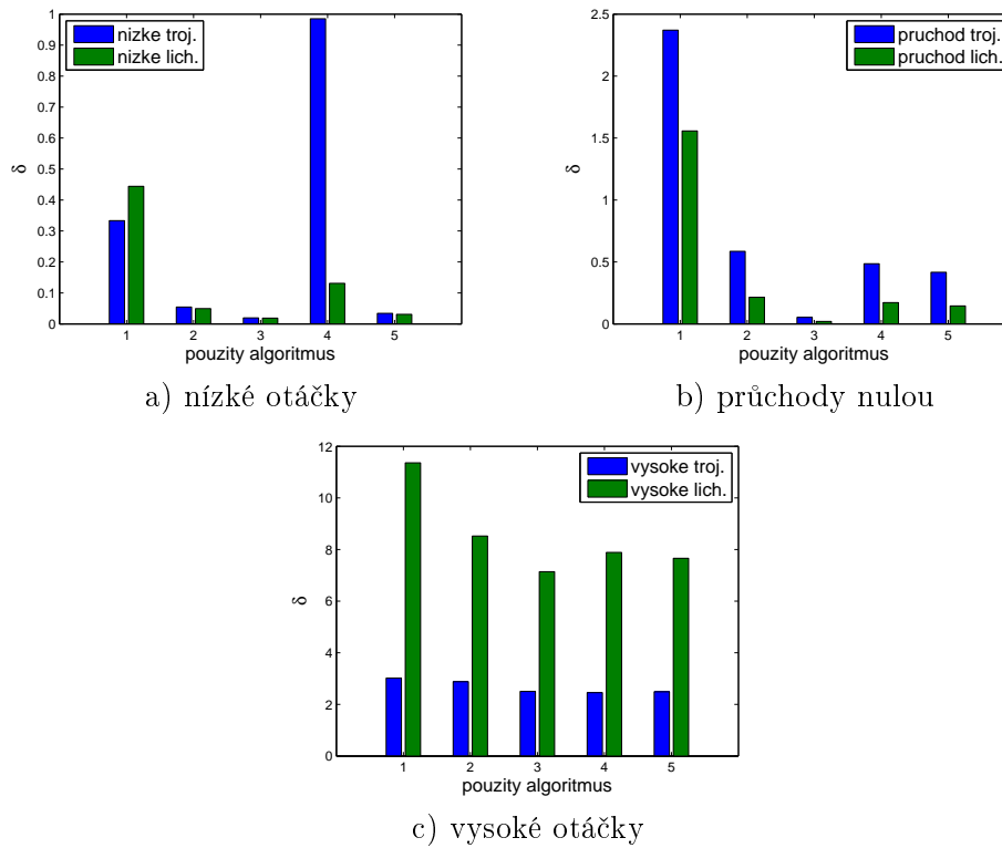
Obrázek 4.14: Dosažené hodnoty středních kvadratických chyb \delta pro profily nízké otáčky a), průchody nulou b) a vysoké otáčky c). Použité algoritmy jdou v pořadí: 1 – vektorové PI řízení, 2 – vektorové LQ řízení, 3 – jednoduchý injektážní návrh, 4 – bikriteriální metoda a 5 – algoritmus využívající hyperstav.
