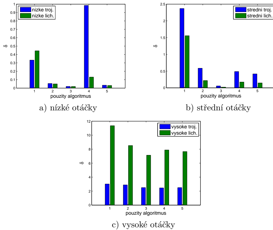
Obrázek 4.14: Dosažené hodnoty středních kvadratických chyb \delta pro profily a) nízké otáčky , b) střední otáčky a c) vysoké otáčky . Použité algoritmy jdou v pořadí: 1 – PI, 2 – LQ-CE, 3 – INJ, 4 – BK a 5 – LQ-HS.
