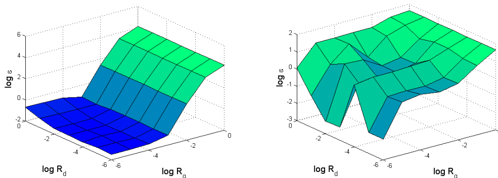
Obrázek 4.3: Posouzení vlivu matice R na velikost střední kvadratické chyby. Vlevo je zachycen výsledek jednoduchého modelu při užití referenčního profilu vysoké otáčky – lichoběžník a vpravo pak výsledek ze simulátoru s profilem střední otáčky – lichoběžník. Všechny osy jsou logaritmické a označení \varepsilon reprezentuje střední kvadratickou chybu.
